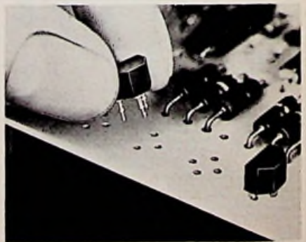
Afb. 6. Het afknippen van draden vervalt bij „lock-fit“ transistoren geheel.
